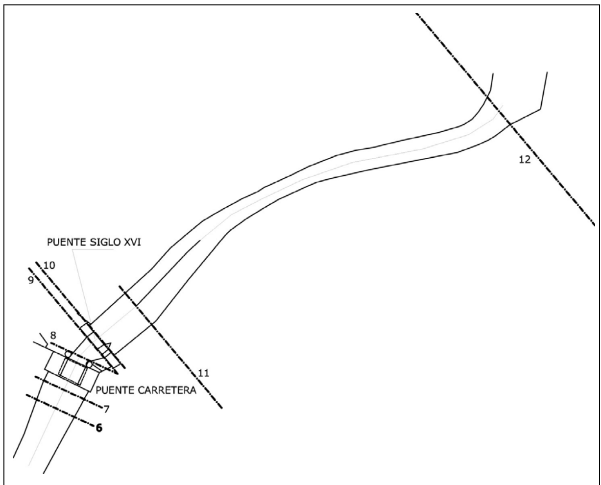
Planta de situación de los puentes y las secciones
