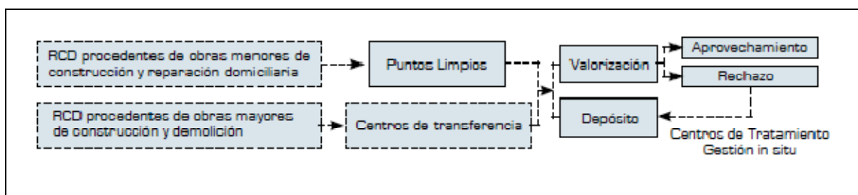
Figura 3.- Esquema de gestión de RCD
