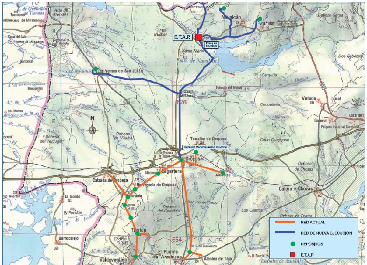
Figura 5.- Obras previstas en el II Plan Director de Abastecimiento
